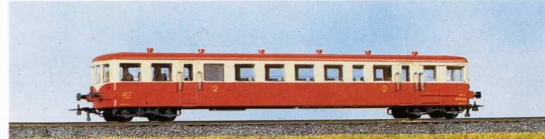
AS (Société l'Emboutissage) Einheitsbeiwagen mit kleinem Gepäckraum, für Dieseltriebwagen aller Typen, Serie XRBD 8100 der SNCF Diesel railcar XRBD series 81, SNCF
