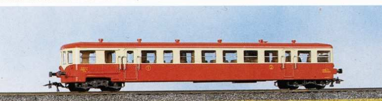
AS (Société l'Emboutissage) Einheitsbeiwagen mit kleinem Gepäckraum, für Dieseltriebwagen aller Typen, Serie XRABD 7300 der SNCF Diesel railcar XRABD series 7300, SNCF
